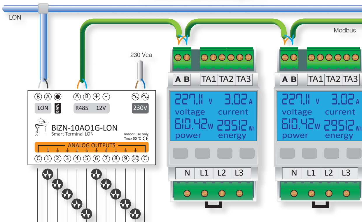
Esempio di schema elettrico con contatori d'energia
